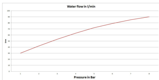
Wasserdurchfluss des Shower head in Abhängigkeit vom Druck.
